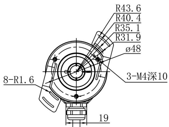
BTS58-H 尺寸图：
